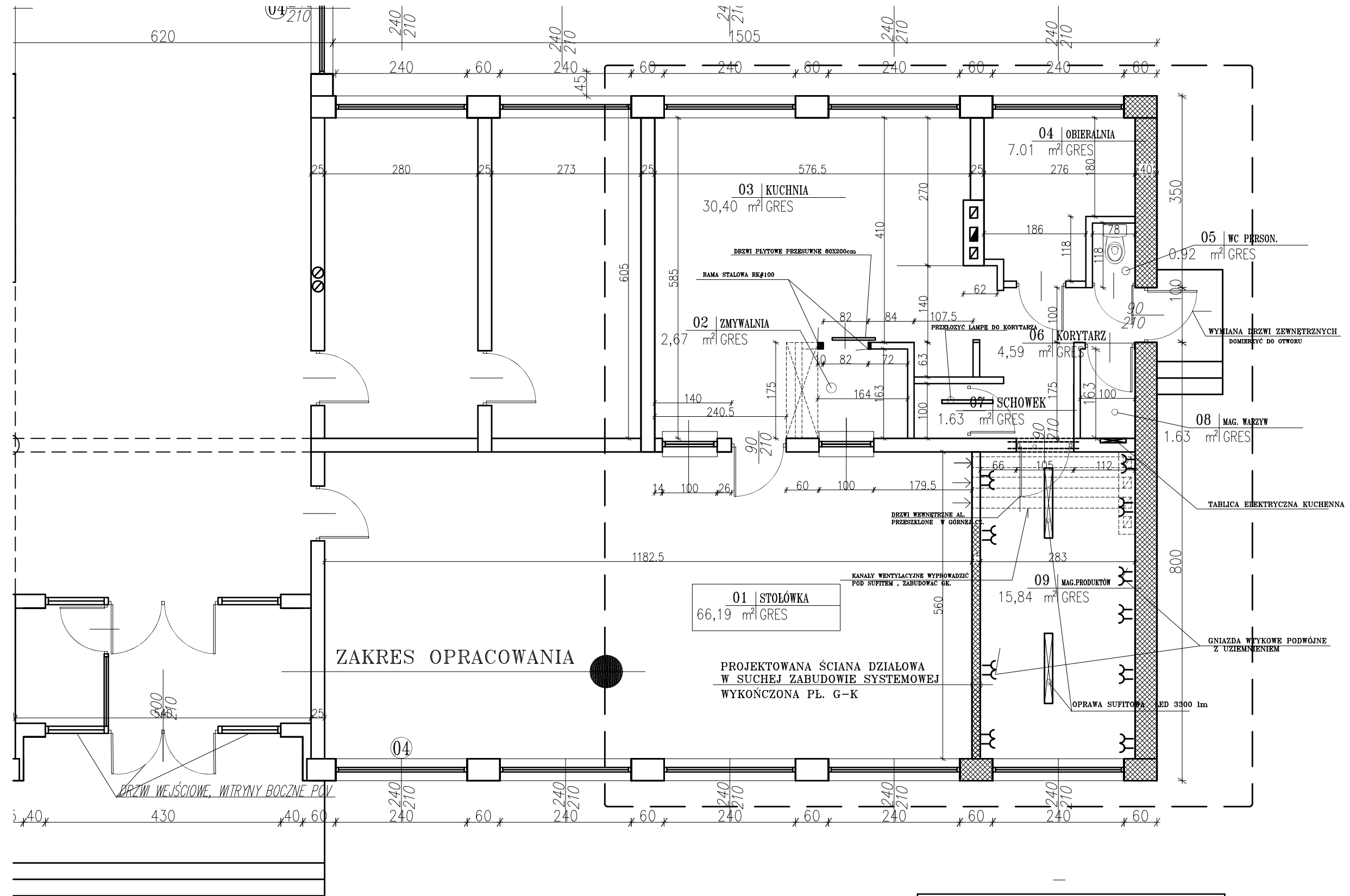
RZUT KUCHNI ZAKRES PRZEBUDOWY INSTALACJA ELEKTRYCZNA SKALA 1:75
