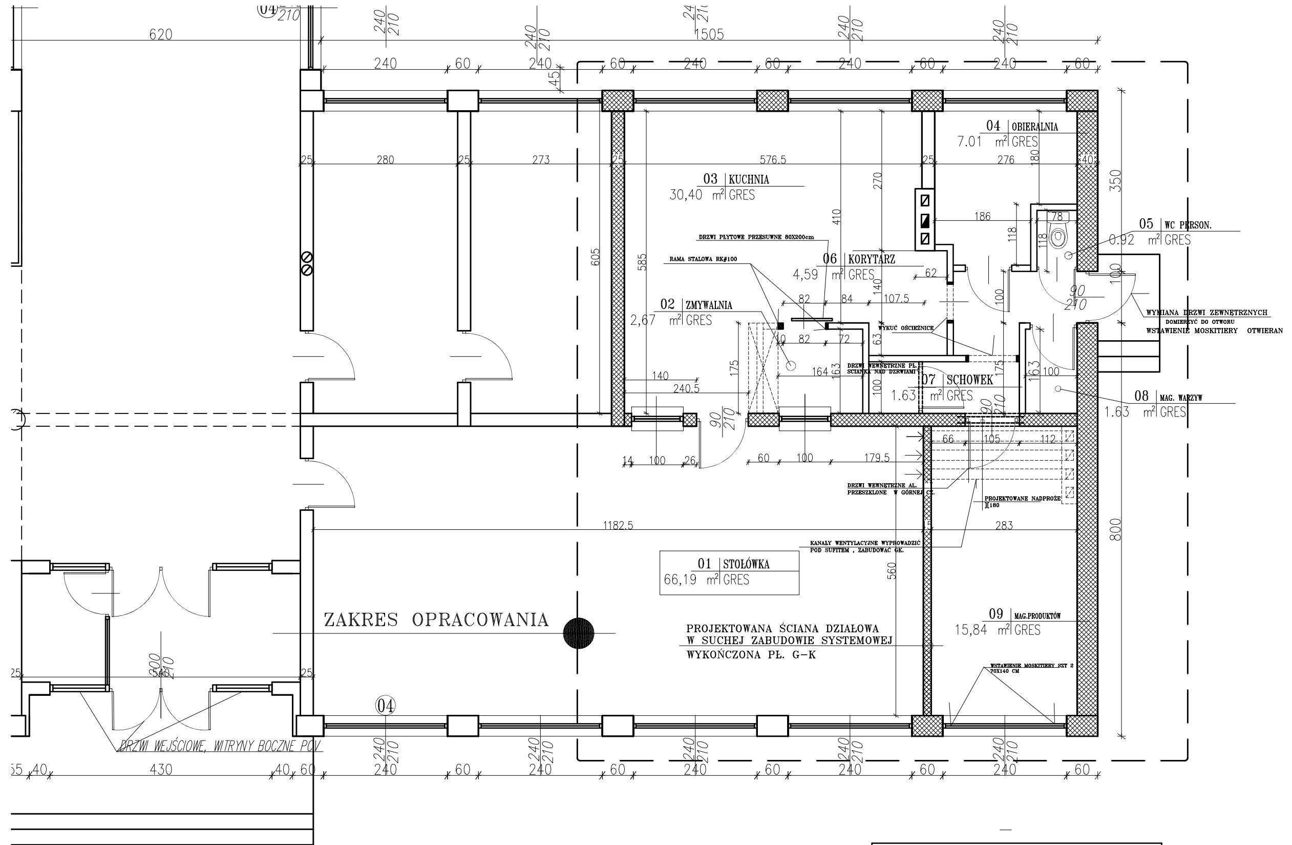
RZUT KUCHNI ZAKRES PRZEBUDOWY SKALA 1:75
