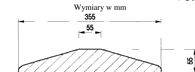
KSZTAŁT I WYMIARY W PRZEKROJU POPRZECZNYM PRZYKŁADOWYCH PROGÓW PODRZUTOWYCH (wg [23])
