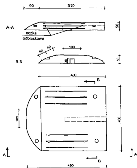
Rys. 3. Próg typu listwowego długości 900 mm i wysokości
