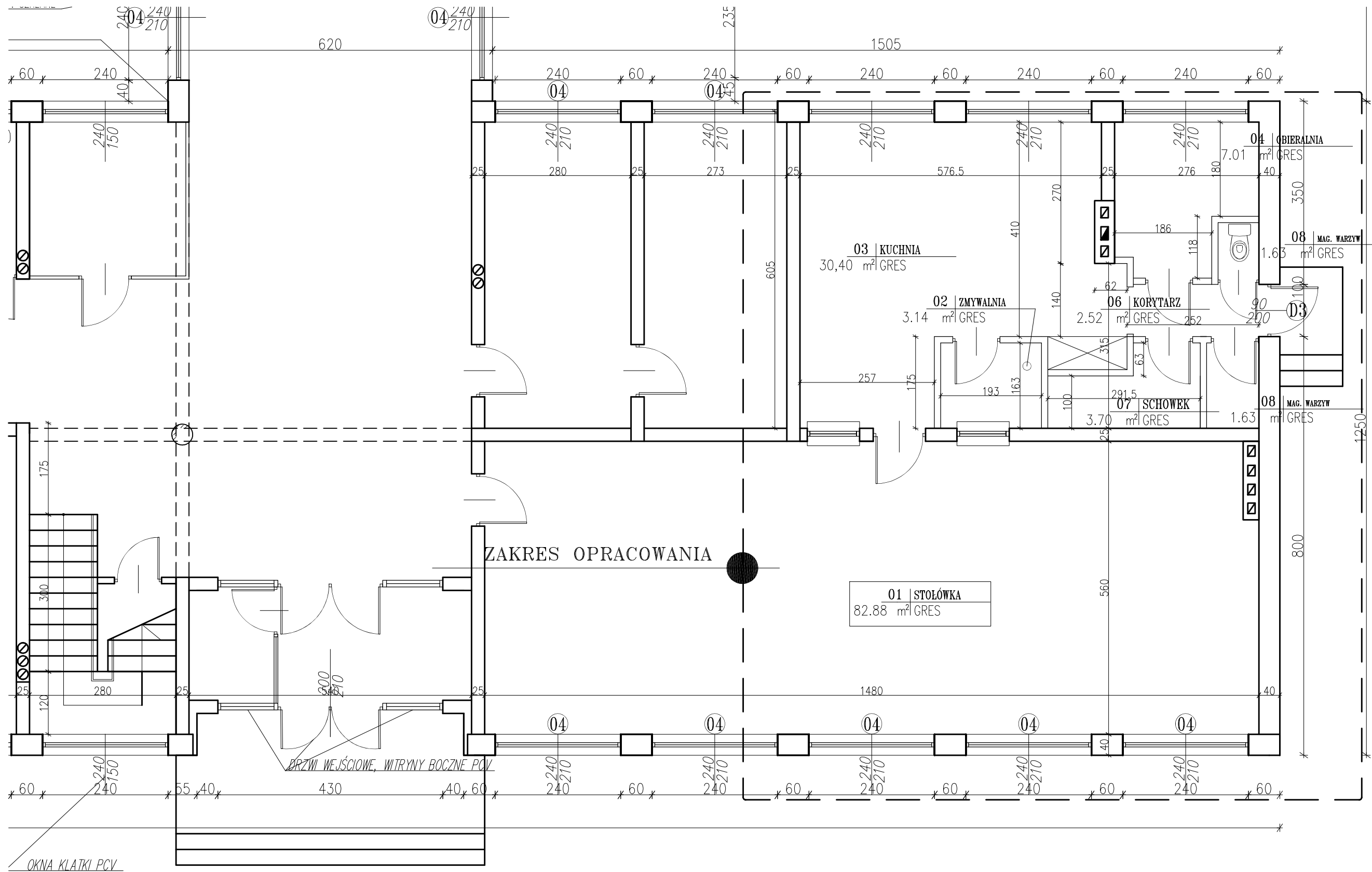
RZUT KUCHNI STAN ISTNIEJĄCY SKALA 1:75
