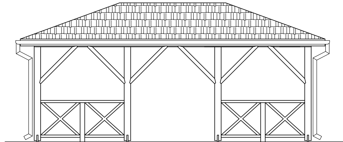
ELEWACJA WEJŚCIOWA
