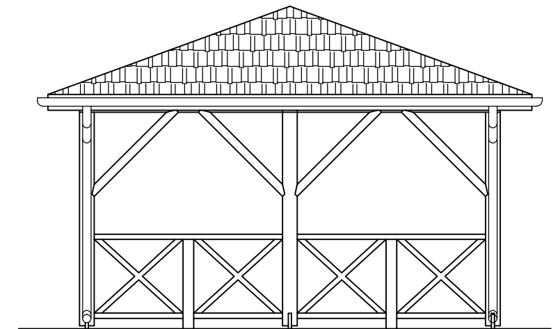
ELEWACJA BOCZNA
