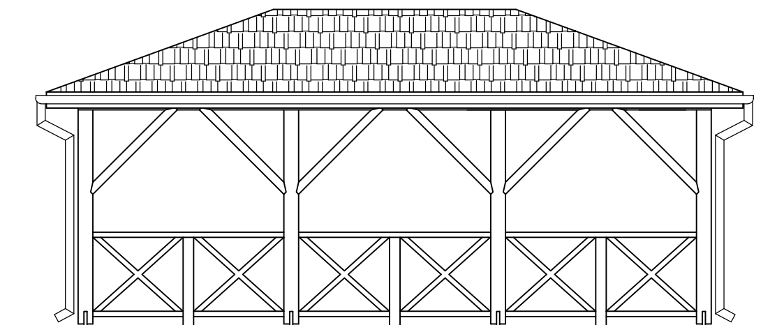
ELEWACJA TYLNA
